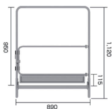
妻面手摺(開閉)
